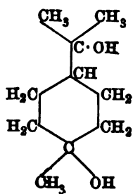
cis-Terpin.
